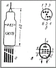
Рис. 41. Лампа 1Ж17Б: а — основные размеры; б — вид на цоколь со стороны выводов; в — схематическое изображение; 1 — катод, нить накала (плюс); 2 — катод, нить накала (минус); 3 — экран (подключается к общему минусу); 4 — третья сетка; 5 — вторая сетка; 6 — первая сетка; А — верхний вывод на баллоне — анод.
